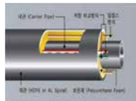
이중보온관
