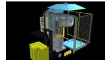
전기식 래들예열장치
